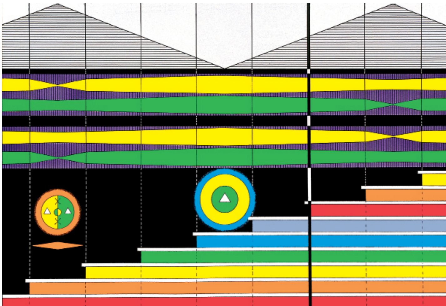
Polprincippet kosmiske kredsløb
